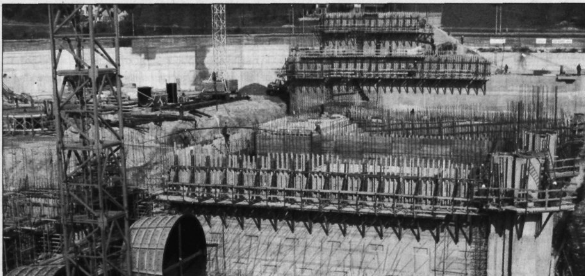
Prvi od treh konusov je že »skrit« v betonu, v ozadju prvo prelivno polje
