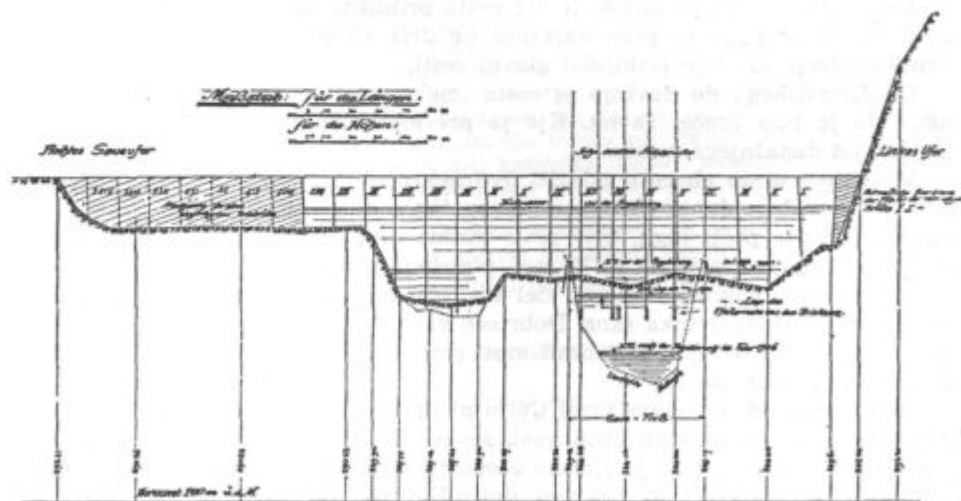
Trloris in profil lesenega mostu v Črnučah (po Schmidu)
