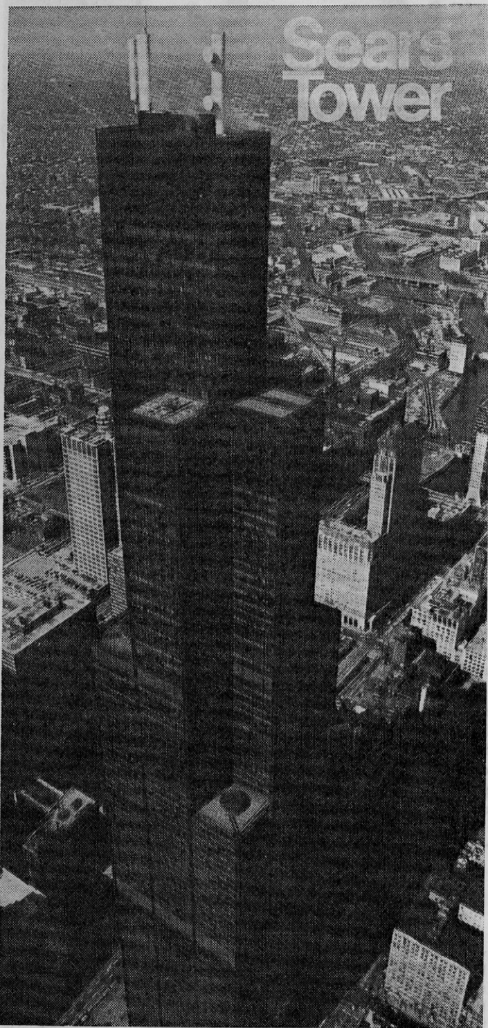
Poslovna stolpnica (Sears Tower) je 110-nadstropna zgradba, katera meri v višino 443 metrov in je v svoji izgradnji zahtevala dobo štirih let. Ogrodje stolpnice je sestavljeno iz 76.000 ton jekla, iz 16.000 oken; medtem ko 114 kamnitih kesonov podpira 222.500-tonsko zgradbo.
