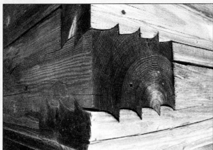
Povezave (spone) s četvernim lastovičjim repom
