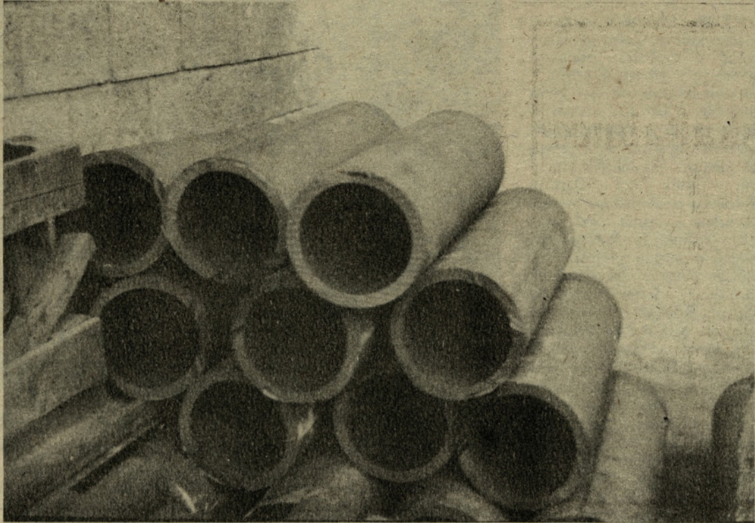
DRUGI NA SVETU – Pred kratkim je v TOZD Livame Ferralita stekla proizvodnja kontinuirano vlečenih cevi na novi napravi. Z osvojitvijo takšne proizvodnje se Ferralit uvršča med edine tovrstne proizvajalce na svetu, kar mu zagotavlja tudi uveljavitev na mednarodnem tržiču. Na sliki: Odlitki kontinuirano vlečenih cevi premera 300x240 mm.
