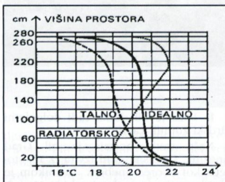
Sl. 1 Temperaturni vertikalni profil v prostoru pri različnih ogrevalih
