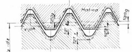
Sl. 9 ISO navojni spoj v prilegu H/g ali h/G
