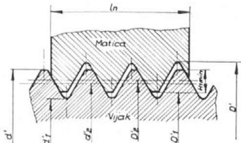
Sl. 7 Navojni spoj na zgornji odnosno spodnji meji tolerančnega polja H/h
