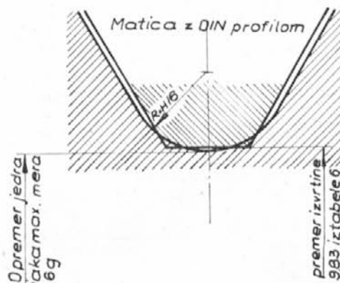
Sl. 15 Prekrivanje ISO in DIN navoj. spoja v mejnem slučaju
