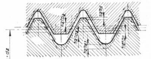
Sl. 10 ISO navojni spoj v prilegu G/g ali g/G
