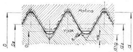
Sl. 8 ISO navojni spoj v prilegu H/h
