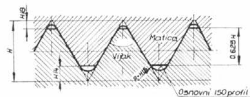
Sl. 4 Profil novega ISO navoja
