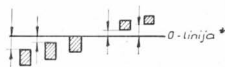
Sl. 11 Položaj tolerančnih polj za navoj vijaka
