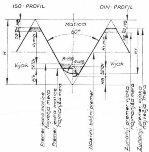
Sl. 5 Primerjava med ISO in DIN navojem
