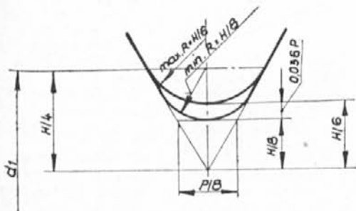
Sl. 13 Mejne vrednosti radiusa dna navoja vijaka
