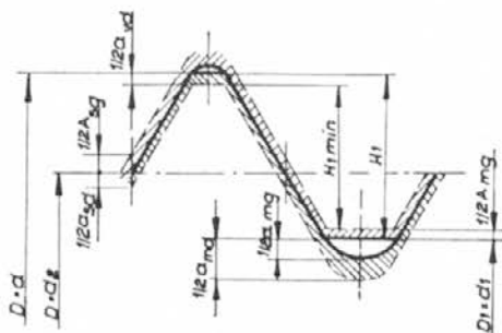
Sl. 6 Nazivni profil ISO navoja v tol. polju H/h
