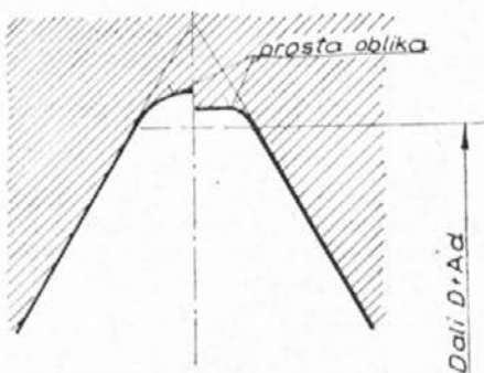
Sl. 14 Oblika dna matičnega navoja
