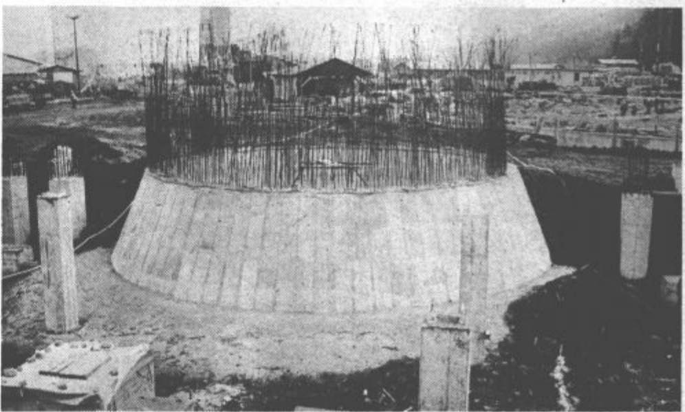
Delavci celjske temeljne organizacije združenega dela Gradis, ki opravljajo gradbena dela, so končali temeljenje dimnika nove Termoelektrarne Šoštanj 4.
