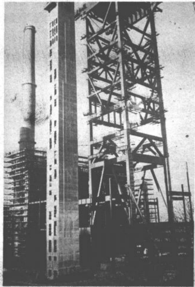
Na gradbišču nove Termoelektrarne Šoštanj 4 bodo sredi meseca decembra končali z deli pri montaži glavne nosilne jeklene konstrukcije kotla; montažna dela izvaja zagrebško podjetje „Braća Kavurić“
