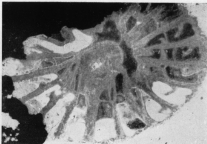
Taf. 7, Fig. 1. Lophophyllidium pendulum var. carinthiaca (Felsler), Querschliiff, \times 10
