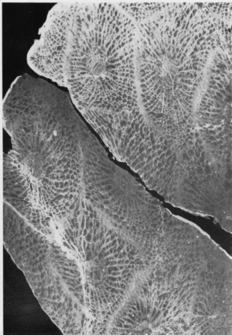
Taf. 1. Wentzellophyllum arminiae (Felsner), Querschliff, \times 5
