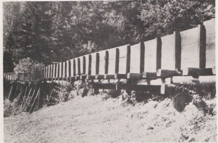
Po zgoraj prepadnih strminah se je vil leseni žleb, zgrajen lepo in estetsko, kot so znali njega dni
