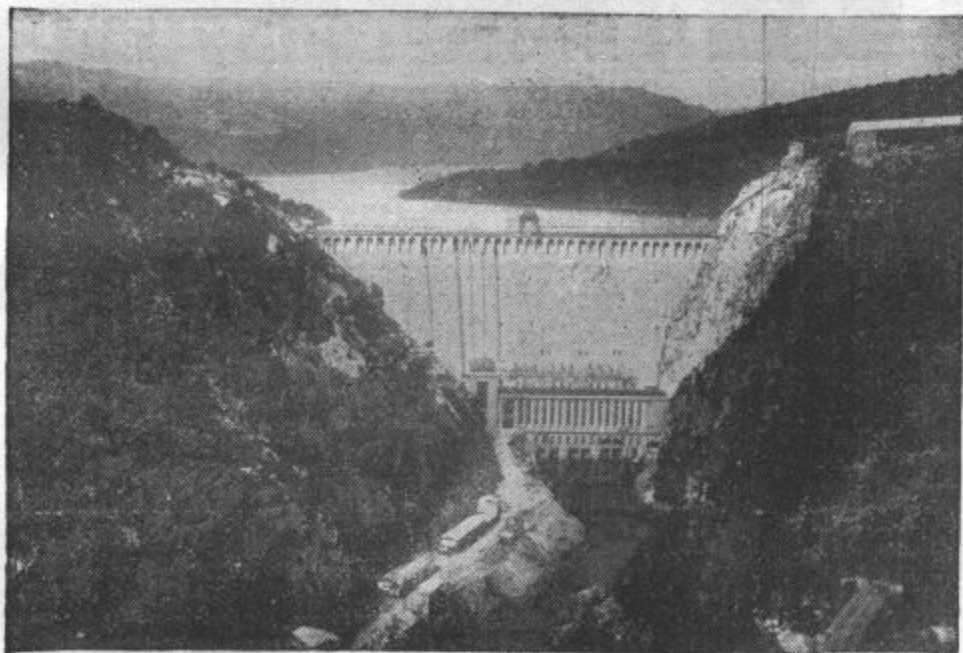
CENTRALA, KI NAPAJA PARIZ Z ELEKTRIKO. Pogled na dolinsko pregrado in električno centralo Sarrens v Centralnem masivu v Franciji, odkoder oskrbujejo z električno energijo Pariz in njegovo okolico. Električni tok prihaja iz te centrale v Pariz pod napetostjo 220.000 voltov. Na centralo je priključeno nad pet milijonov odjemalcev električnega toka.
