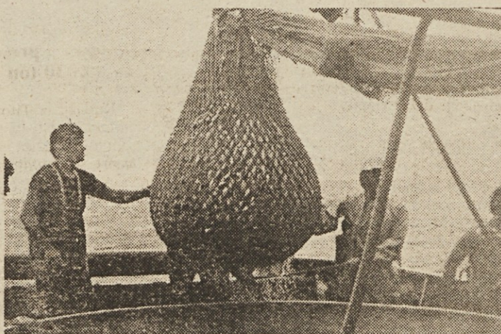
»Droga I«, ladja dvojica naše Droge II. Dolžina 30 m, nosilnost 156 BRT, motor 800 KM, največja hitrost 12 vozlov na uro. Oprema: dva navigacijska radarja, avtopilot, dva ehografa (za sledenje ribjih jat), mreža je »koča«, 150 m dolga, 12 m široka. V ladijsko hladilnico gre do 8 vagonov rib. Posadka: 10 mož.
