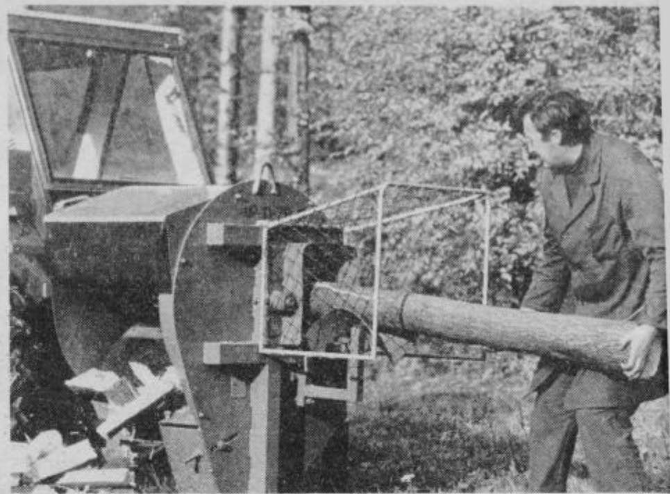
Stroj za pripravo, hkratno sekanje in cepljenje drv Drvar je primeren za razrez lesa s premera 19 centimetrov. Drva lahko razseče na željeno dolžino od 20 do 60 centimetrov montira pa se lahko na hidravlični mehanizem traktorja.
