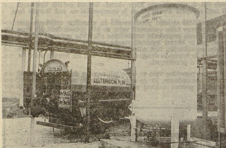
Prvo polnjenje 7.500 l rezervoarja s tekočim dušikom, ki ga bomo uporabljali kot zaščitni plin pri žarenju v novi žarilnici v Železarni Štore. Več o tem v prihodnji številki glasila.
