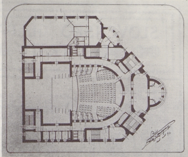
Pritličje
