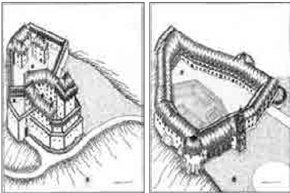
Grad na Gorickem v 15. in 19. stoletju. Aksonometrični študiji (Igor Sapač, 2004).
