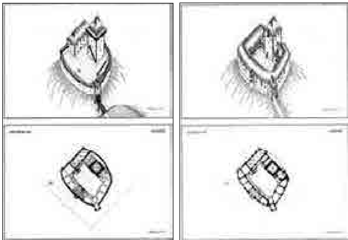
Grad Klevevž na Dolenjskem okoli leta 1396 in 1700. Aksonometrični študiji (Igor Sapač, 2002).
