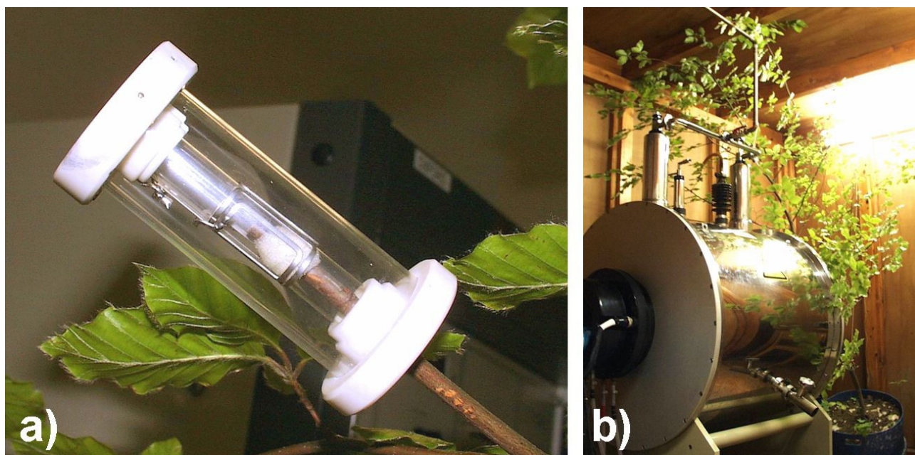
Slika 1: a) Namestitev RF-tuljave na odrezano vejico bukve in b) Buke v laboratoriju med slikanjem. Slikana vejica je skupaj s tuljavo nameščena v odprtino horizontalnega superprevodnega magneta.
