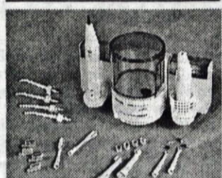
aparatus za nego zob, ROWENTA, MH 670, posoda s pokrovom za 5 dl vode, električna ščetka z eliptičnimi treslji 2500/min
