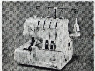
šivalni stroj, ELMA, Elnalock 614, enostavno rokovanje in dobra kakovost, štirinisti in dvoigeln elektronski stroj z diferencialom, možnost šivanja dvo-ali trinitno, število šivov 6+3
