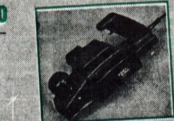
oblič, BLACK&DECKER, KW 750, moč 500 W, 15000 vrt/min, globina reza 0-1,5 mm, širina reza 75 mm
