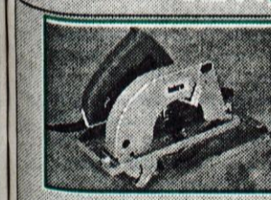
krožna žaga, ISKRA ERO, KZ 55 D, moč 830 W, 4300 vrt/min, globina reza 50 mm
