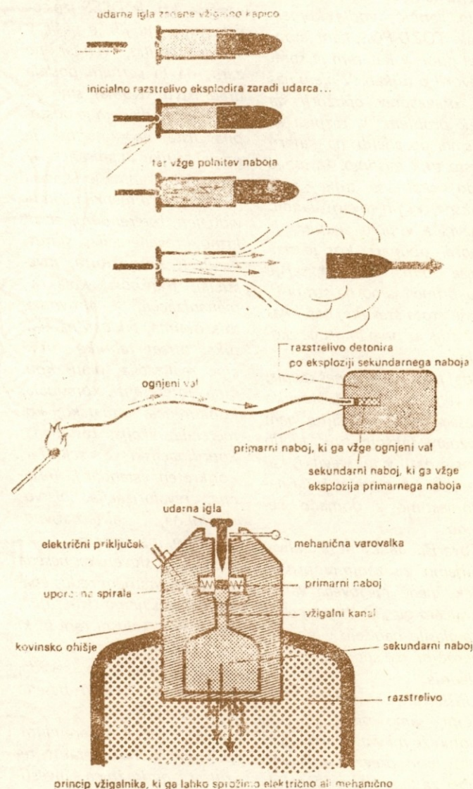
Princip vžigalnika, ki ga lahko sprožimo električno ali mehanično
