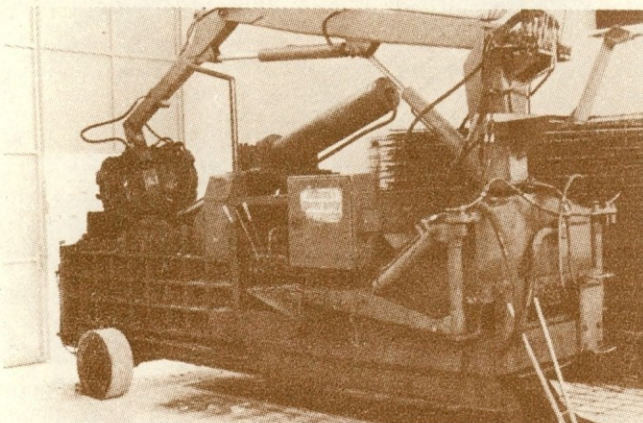
Stiskalnica za jeklene odpadke „S-12“, ki so jo Jeseničani dobili iz Brežic.
