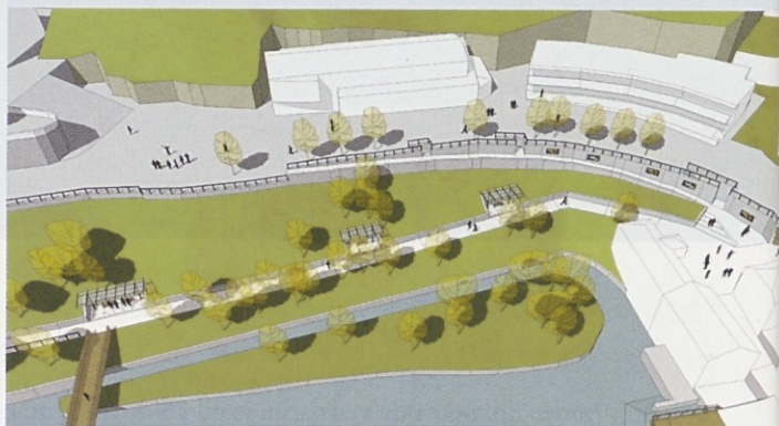
Slika 2 Vizualizacija mostu in nove dostopne poti mimo Modrijanove domačije.
