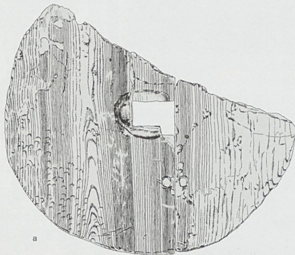
Risba kolesa. Notranja (a) in zunanja (b) stran s preseki. Narisal: T. Korošec
