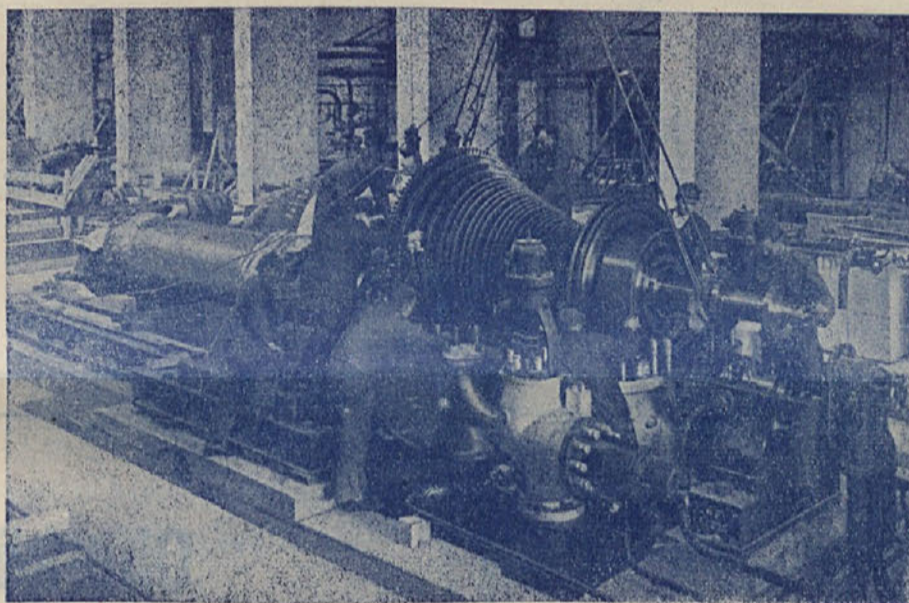
Montaža 20.000-kW turbogeneratorja
