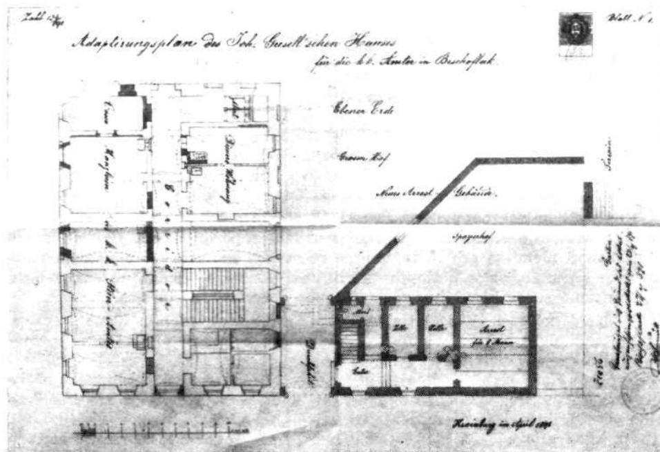
Načrt za adaptacijo stavbe in za gradnjo prizidka iz leta 1891
