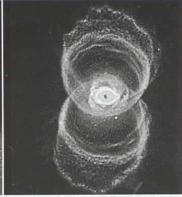
Vesoljski teleskop Hubble, ki kroži v višini 593 km nad Zemljo s hitrostjo 28.000 km na uro. Objavljamo tri njegove fotografije iz vesolja: Desno : Meglica Hourglass, oddaljena 8.000 svetlobnih let ( Glej spodaj )
