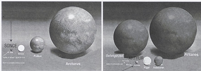
Levo: Zvezda Arthur (največja) v primerjavi z velikostjo našega Sonca Desno: Zvezda Antares (največja) v primerjavi z velikostjo zvezde Arthur
