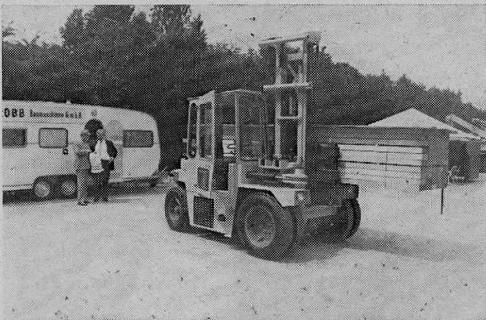
Stranski viličar, ki ga je mogoče takoj spremeniti v čelnega
