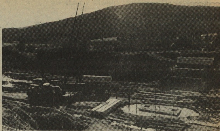
Nadvoz 4-01. Razpetina med obrežnima opornikoma bo nekaj nad 50 metrov; konstrukcijo bodo podpirali še trije pari stebrov, ki jih je voz-nik SPO prav na dan nastanka fotografije pripeljal iz OGP in so jih iste-ga dne na gradbišču tudi vgradili. Prek avtoceste bo po tem nadvozu, v blagem naklonu, speljana cesta v Vel. Ubeljsko.
