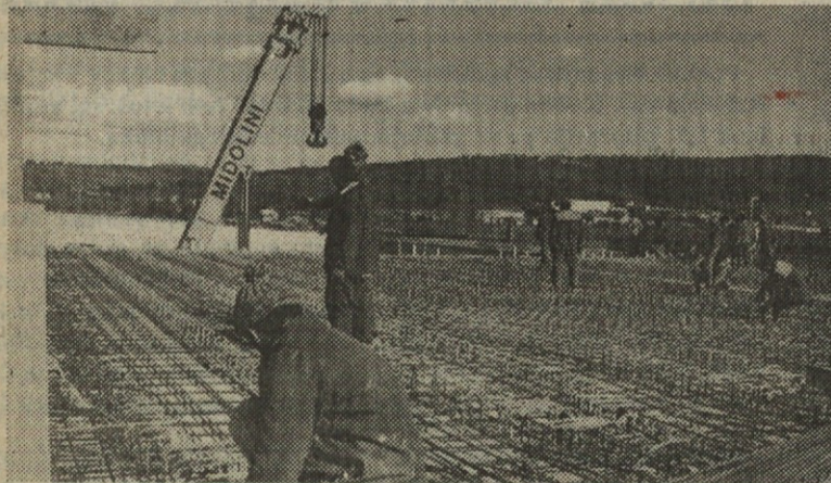
Polaganje in vezanje armature za ploščo nad že zmontiranim delom nadvoza Bivje, po katerem bo progo prečkala bodoča avtocesta.
