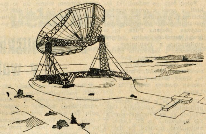
2. Podoba novega, v vseh smereh gibljivega radijskega teleskopa, ki ga gradijo pri Jodrell Banku v Sheshiren, Anglija.
