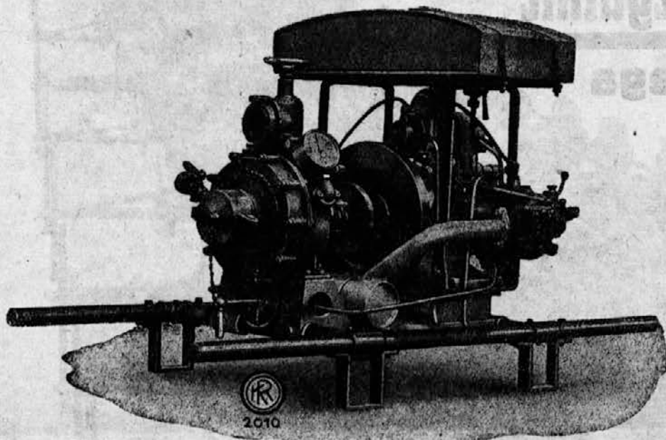
Motorna brizgalna tipa „MB2“.
