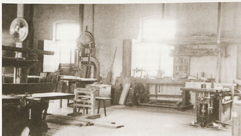
Mizarska delavnica Karla Jevščeka je bila ena redkih, ki je bila že pred 1. svetovno vojno opremljena s stroji. Pred 2. svetovno vojno je bila prenovljena, opremlili so jo tudi z več novimi stroji. Na desni je mizni rezkar, ob oknu stružnica in orodje, ki ga je uporabljal strugar, levo ob oknu tračna žaga, skrajno levo pa poravnalnik. Nad njim visi rezilo za vzdolžno žaganje (foto: arhiv družine Jevšček).
