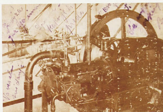
Pogonski bencinski stroj pod strojno delavnico Karla Jevščka leta 1910. V ozadju je viden jermenski pogon, vezan na bencinski stroj v ospredju, ki je poganjal preostale stroje. Razglednica je iz arhiva družine Jevšček in je bila poslana 23. junija 1915.
