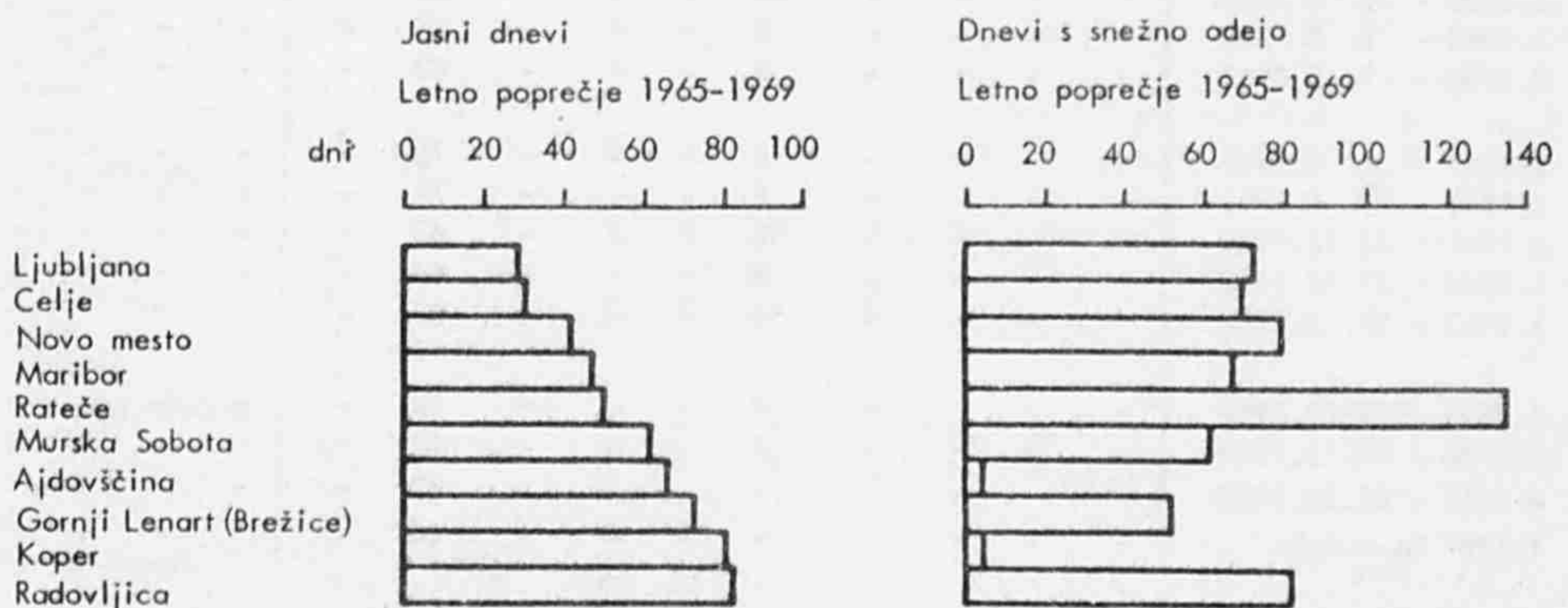
GRAF. 1-2. ŠTEVILO JASNIH DNI IN DNI S SNEŽNO ODEJO
