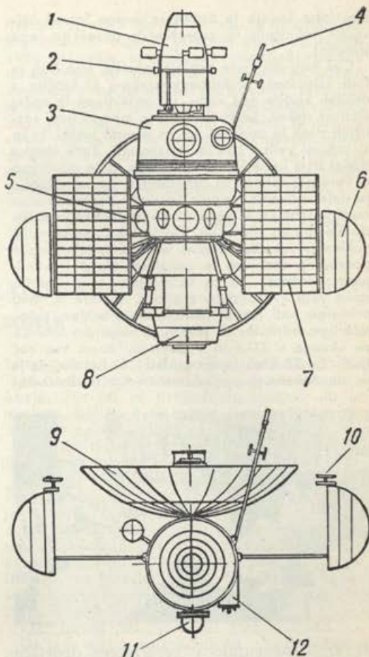
Sl. 7: Očrt sovjetske vesoljske sonde »Venera 3«, ki se je spustila na Venero. Stevilke pomenijo: 1 — pomožni motor, 2 — mikromotorji za usmerjevanje, 3 — glavna kabina, 4 — antena magnetometra, 5 — orientacijski sistem, 6 — radiatorji za toplotno regulacijo, 7 — paneli s sončnimi celicami, 8 — odsek z merilnimi napravami, 9 — antena z ozko usmerjenostjo, 10 — široko usmerjena antena, 11 — dajatelj za zvezdno in sončno orientacijo, 12 — usmerjevalec k Soncu.
