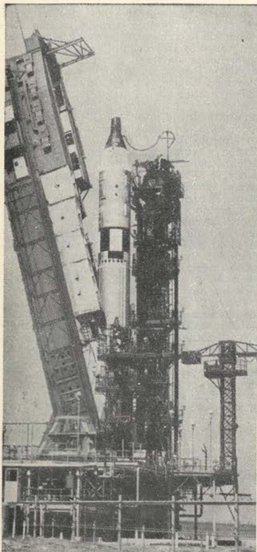
Sl. 1: Naprava za izstrelitev kozmične ladje »Gemini«. V središču je raketa vrste Titan, v njeni konici pa kozmična ladja z obema kozmonavtoma. Slika je posneta v oporišču Cape Kennedy v Floridi (ZDA).
