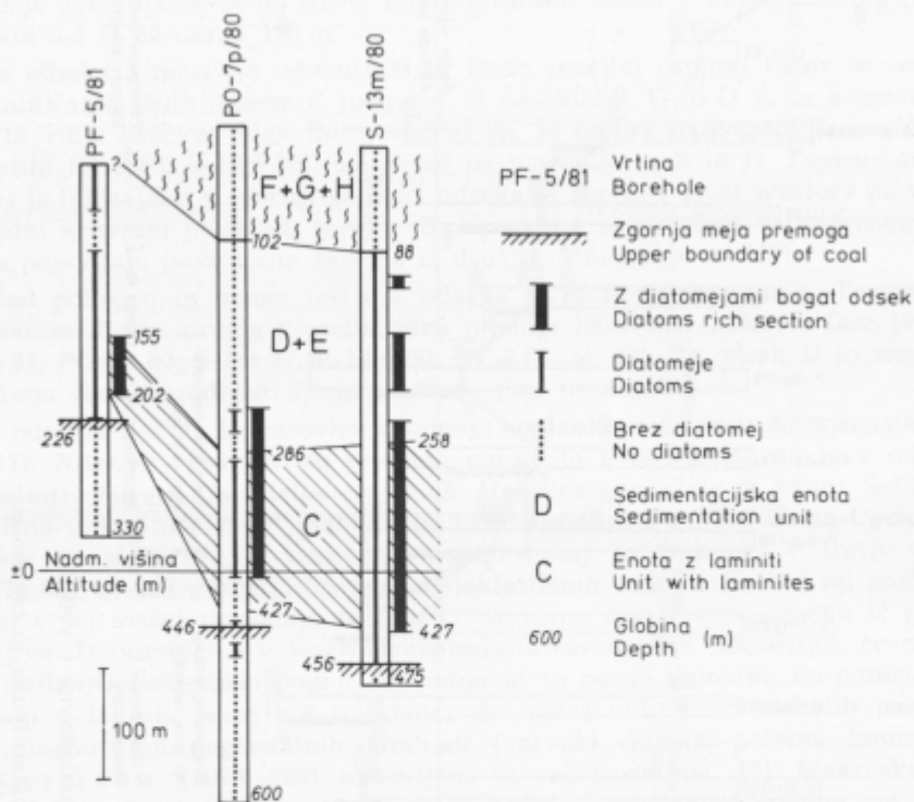
Sl. 11. Položaj diatomej v vrtinah
