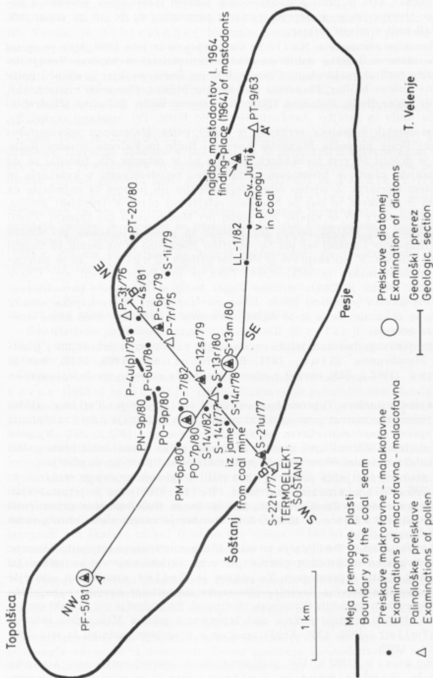
Sl. 1. Položajna karta raziskanih vzorcev
