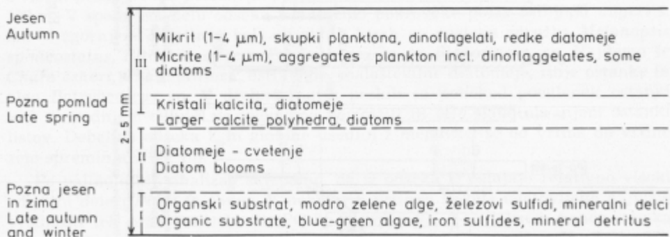
Sl. 12. Sestava jezerske neglacialne varve (prirejeno po Lermanu, 1978, 309). I—III faze sedimentacije v enem ciklu
