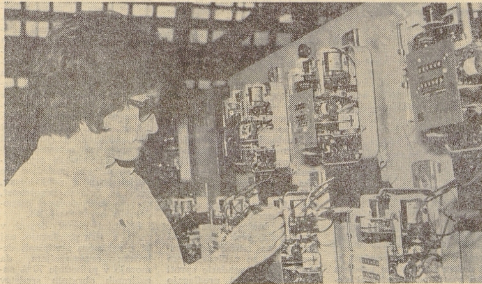
Elektromehanika: na trgu je vedno večje povpraševanje po trifaznih dvotarifnih števcih
