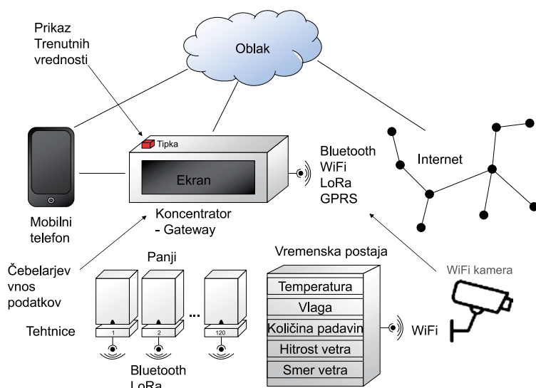
Shema čebelarke nadzorne naprave
