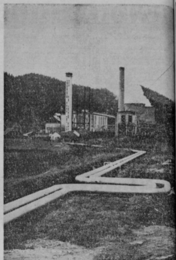
V Soštanju montirajo osnovo nove termoelektrarne železno konstrukcijo, na katero bodo obesili kotel. Visok betonski stolp za dvigalne naprave je že nared, kotel pa bodo »obesili« na pomlad.
