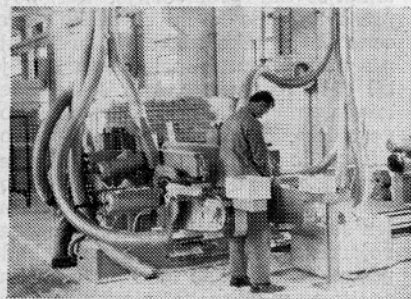
Druga faza v delovnem procesu se opravlja na dvojni čeparki.
