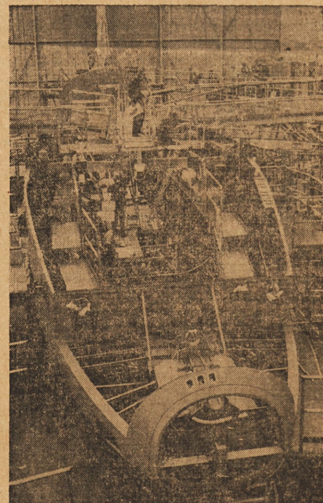
ZA VESOLJSKE POLETE — Vesoljski čolnici bo v prihodnjem desetletju služil za polete v vesolje, predvsem za vzdrževanje zvez med Zemljo in vesoljskimi raziskovalnimi središči ter postajami. Na sliki vidimo graditev tega "čolnica" v vesoljskem oddelku Rockwell International v Palmdalu, Kalif.
