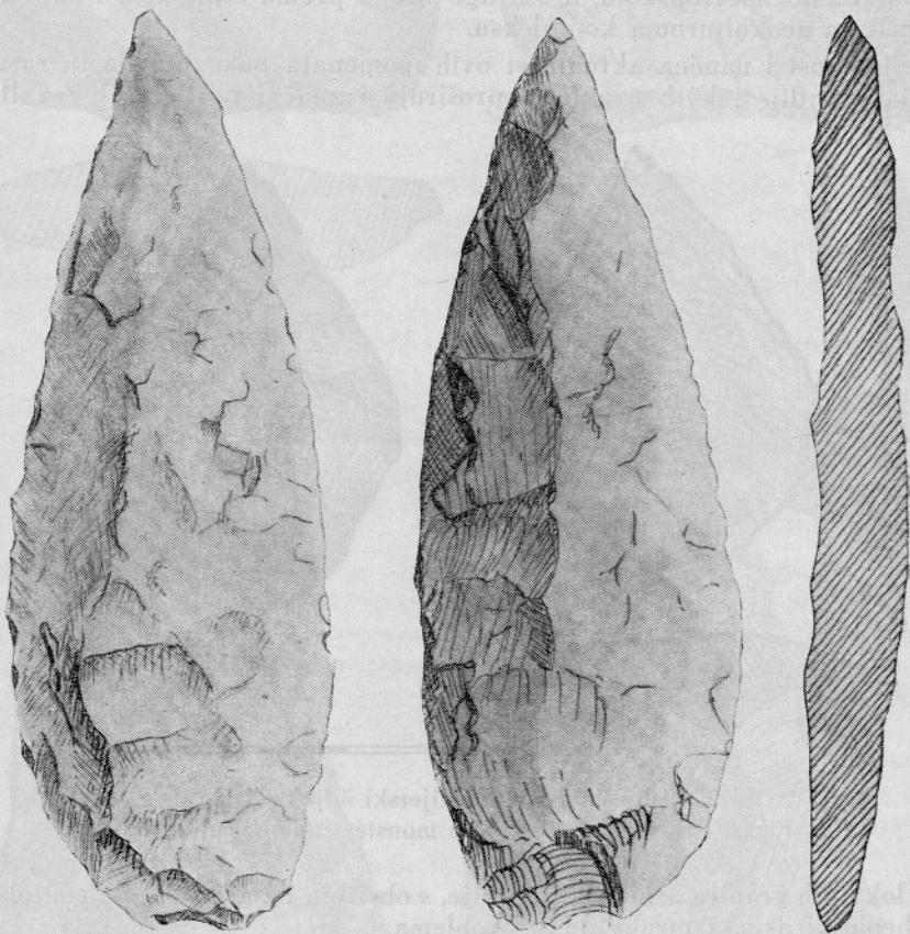
Sl. 5. Risovača 1956: dvostruko obrađeni šiljak. Nar. vel.
