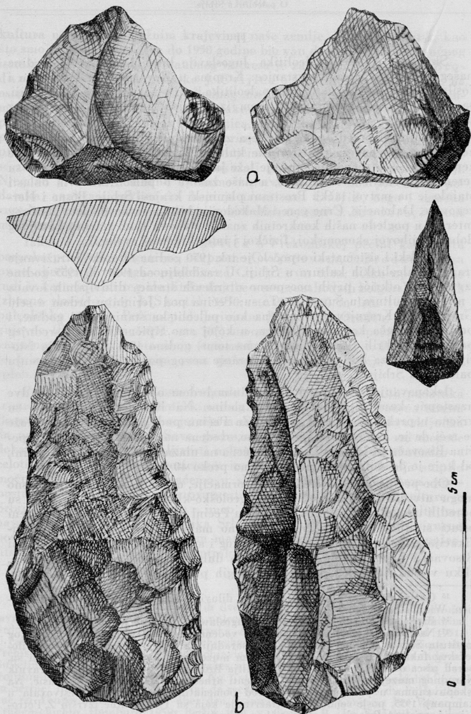
Sl. 1 a. Gradac 1951: trougaoni šiljak. Nar. vel. — 1 b. Gradac 1952: izduženi strugač. Nar. vel.
