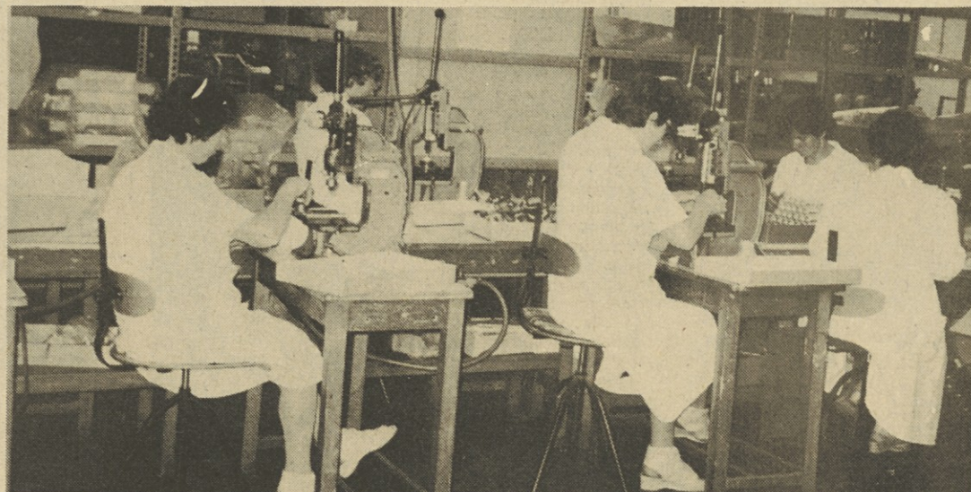
Tudi ta del ročne proizvodnje elektrolitskih kondenzatorjev večjih dimenzij bo treba kmalu zamenjati z avtomatiziranimi linijami.
