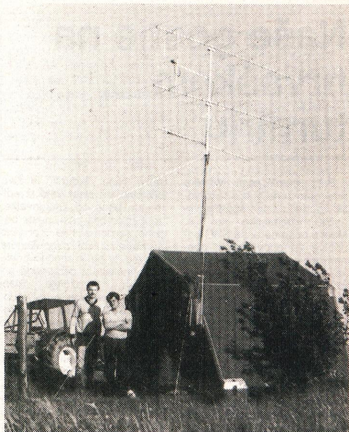
Člani Radiokluba na Trebelniku nad Zavrhom (Kota 807). Lepo je vidna 20 el. antena za 144MHz YUOB in 13 el. za 432 MHz »HOME MADE«
