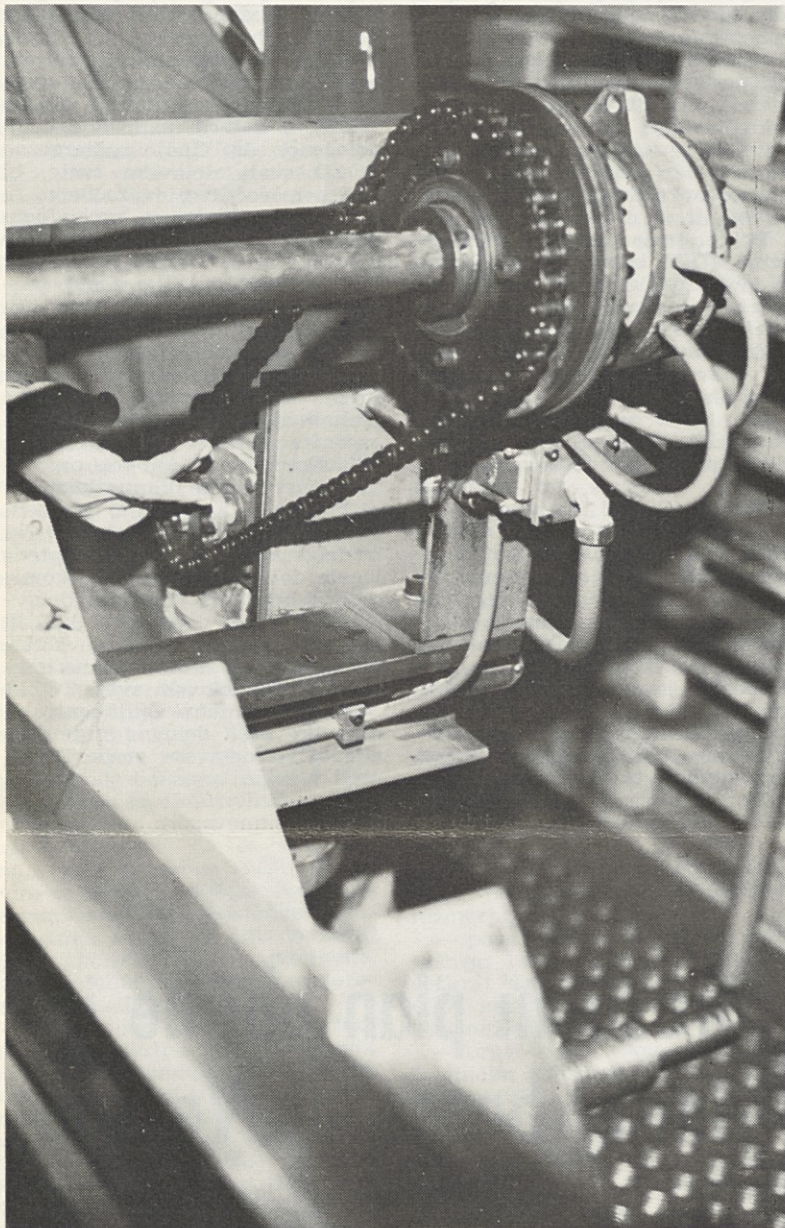
Vsokršni verižni pogon je lahko zelo nevaren, če pazljivost ni zadostna. (Na sliki: rekonstrukcija obratne nezgode pri zavijalnem stroju.)
