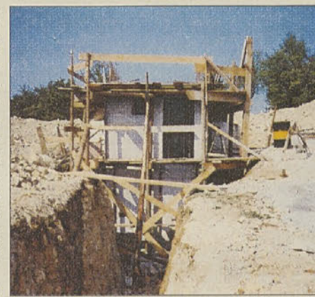
Gradnja rezervoarja 100 m 3 na Rihpvcu v letu 2001
