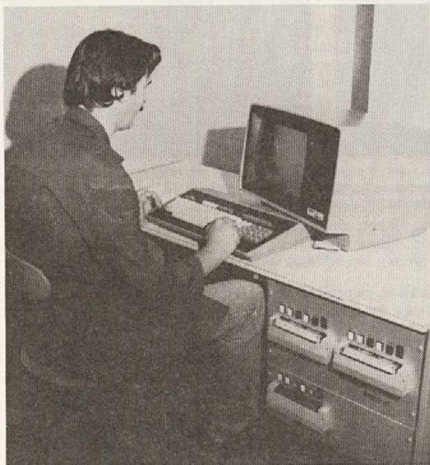
KOREKTURNA NAPRAVA »VIDEOSET« – po reviziji opravi korekturno delo fotostavec-perforist
