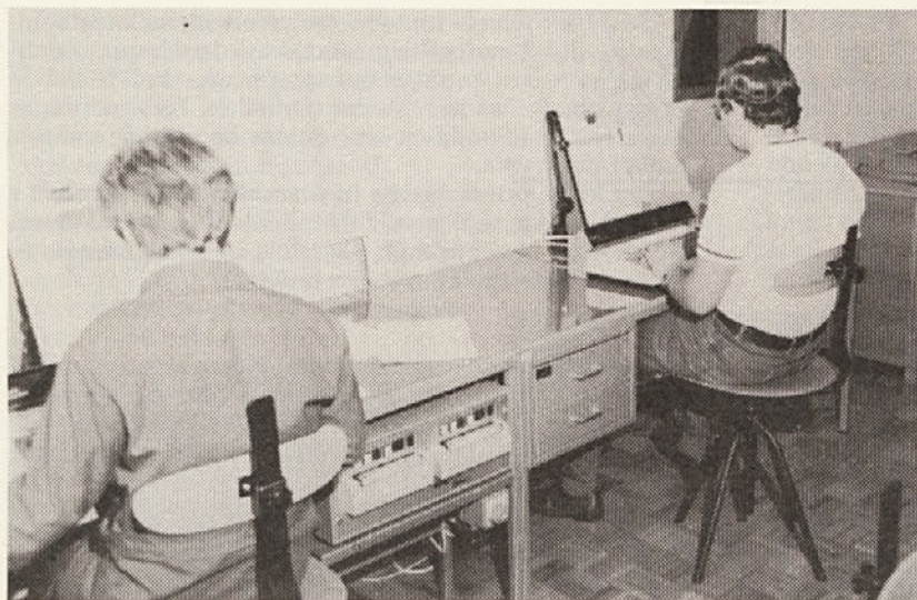
Tipkalna naprava KEY SET-30 v fotostavnem sistemu z držalom za rokopis, ekranom, ki prikazuje zadnjih 32 tipkanih znakov in perforatorjem, na katerem uporabljamo magnetni trak. Na teh napravah delajo fotostavci-perforisti
