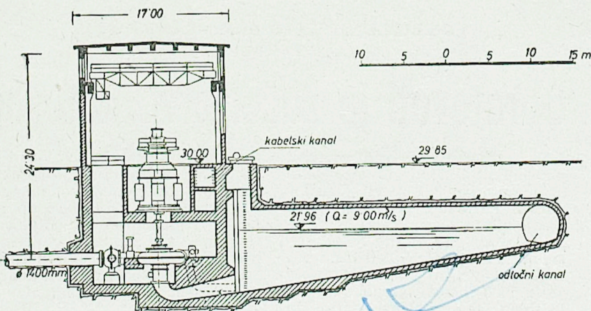
Skica prikazuje prečni rez skozi strojnico bodoče HE Koper. Na levi vidimo konec tlačne cevi s kroglastim zasunom, ki dovaja vodo v Francisovo turbino. Nad njo je generator, ki leži poglobljeno, pokriva ga pa poslopje centrale. Izpod turbine odvaja sesalna cev izrabljeno vodo v odtočni kanal in po njem v reko Osp
