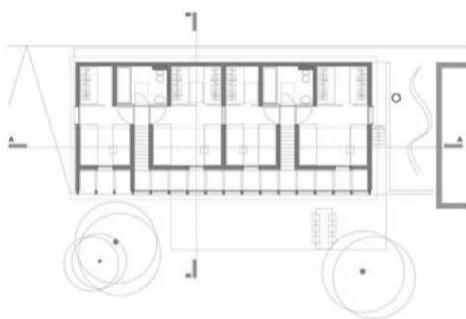
Tloris nadstropja
