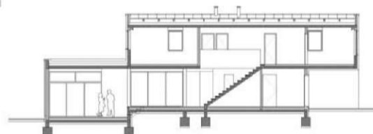
Prerez
