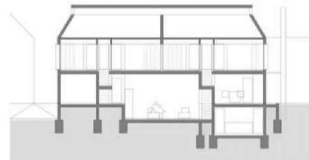
Prerez
