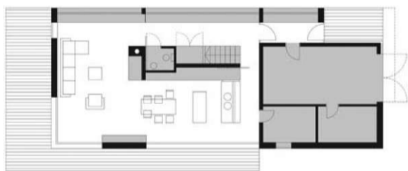
Tloris pritličja
