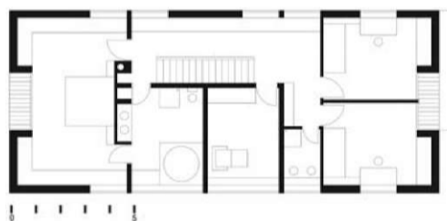
Tloris mansarde
