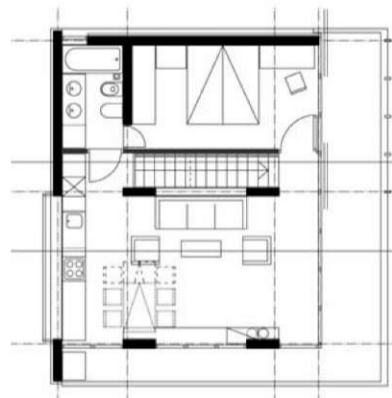
Tloris pritličja
