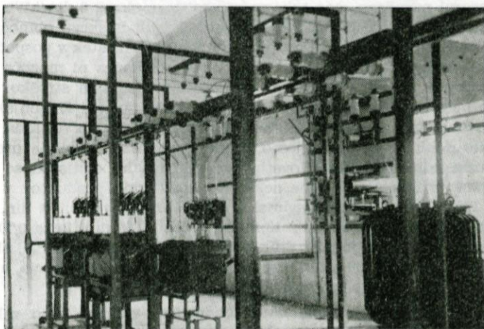
Pritličje transformatorske postaje Grosuplje
