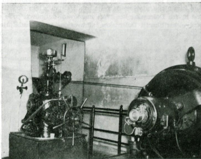
HE Zagradec — Generator št. 2
