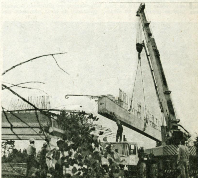
Graditev mostu čez Kamniško Bistrico je hitro potekala in na sliki vidimo železobetonski nosilec za novi most
