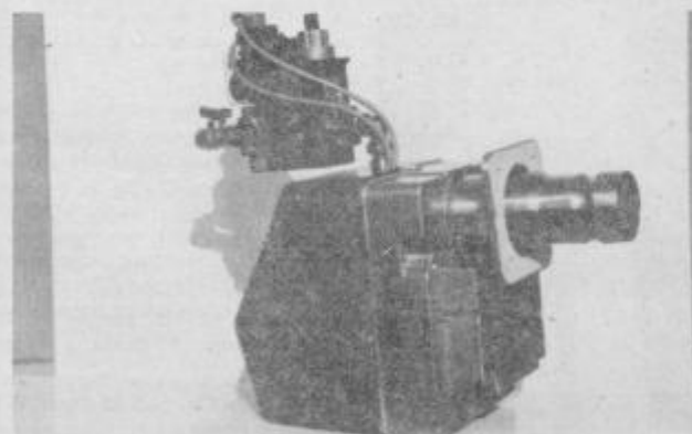
Plinski gorilnik P1, 11-40 kW
