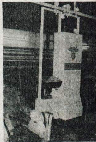
"Krvavi mojster" - naprava za avtomatsko, računalniško vodeno dodajanje močnih krmil. Naprava dodaja krmila po potrebi tudi do desetkrat na dan in je računalniško povezana s kmetovim stanovanjem. Strokovnjaki poudarjajo, da veliko prispeva k večji prirerji in boljši gospodarnosti.
