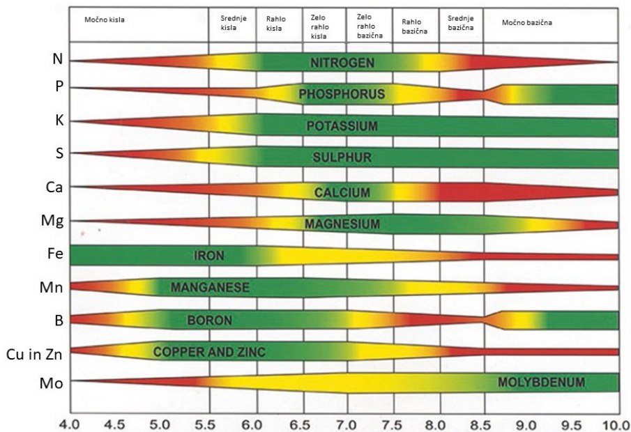
Slika 48: pH-vrednosti, ki prikazujejo vpliv kislosti tal na dostopnost različnih mineralov. Različne barve predstavljajo dostopnost posameznega elementa; zelena: dostopen, rumena: slabo dostopen, rdeča: nedostopen
