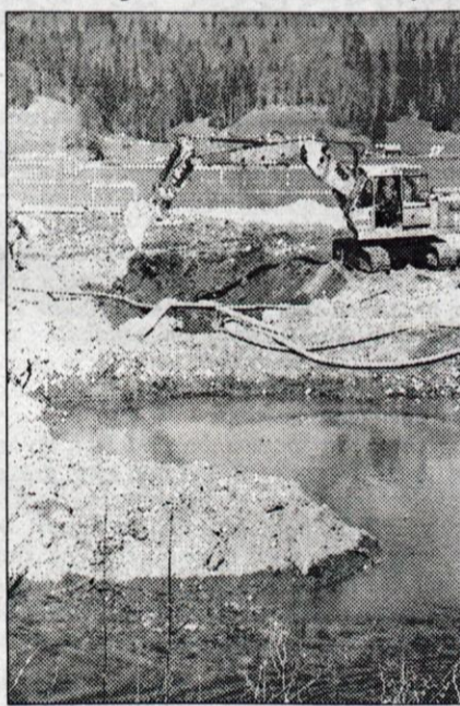
Premoščanje Poljanščice z zbirnim kanalom pri Gorenji vasi.
